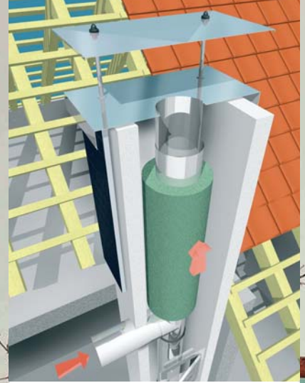
Der LB Universal als Lösung für den Neubau oder die nachträgliche Montage einer Abgasanlage im Gebäude
