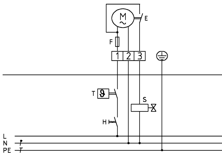
Abb. 6 Anschluss Stellantrieb STA2 (S1)
