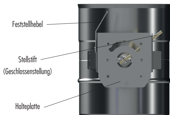
Abb. 1 Halteplatte
