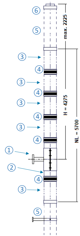
Aufbaubeispiel bis 6,5 m ab oberster Wandbefestigung
