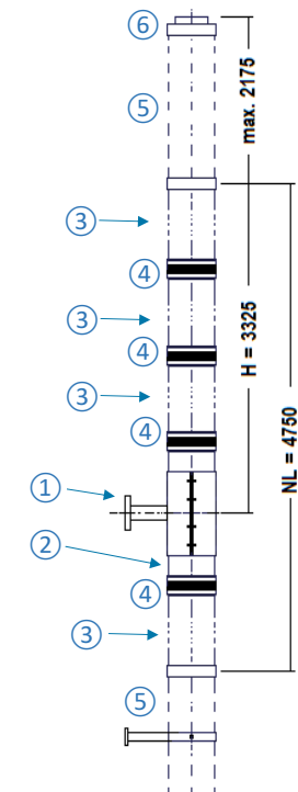
Aufbaubeispiel bis 5,5 m ab oberster Wandbefestigung
