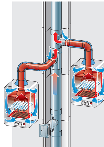
Beispiel für ein LAS-System (raumluftunabhängig)
