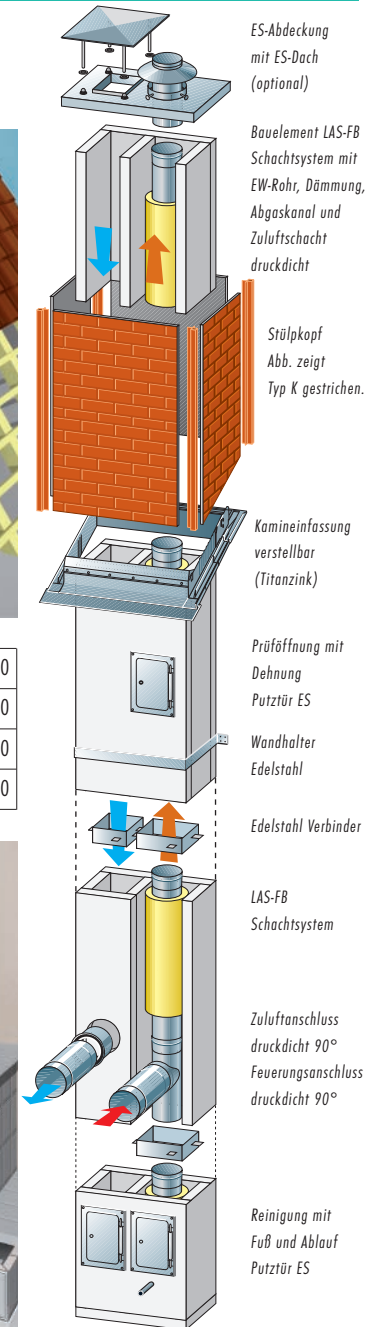
Beispielanbau zweizügig: Abgasführung mit separater Zuluft
