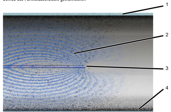
Abb. 13: Funktion Elektrostatische Partikelabscheidung
