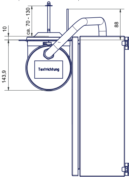
Abb. 7: Maße Ansicht 3 Partikelabscheider Zumikron Outdoor (Draufsicht)
