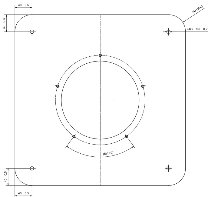
Abb. 14: Maße Anschraubadapter
