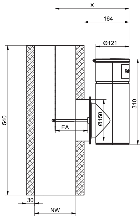
Abb. 7: Maße Ansicht 3 Partikelabscheider Zumikron Outdoor (Draufsicht)
