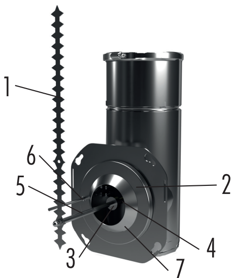
Abb. 18: Elektrode (1), Keramikisolator (2), Verschiebesicherung (3), Elektrodenhalterung (4), Haltestange (5), Thermofühler (6), Strömungskegel (7) Maße Nennweite und Elektrodenabstand
