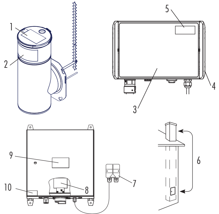
Abb. 4: Beschilderungen Zumikron Outdoor
