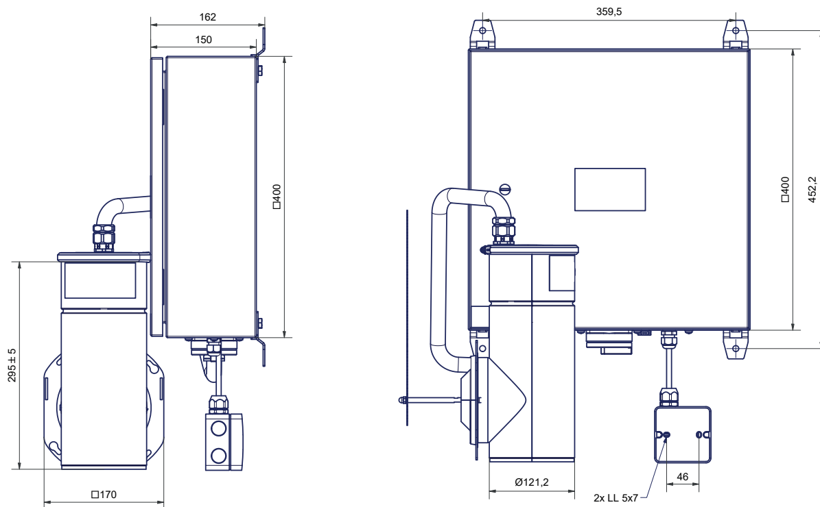
Abb. 5: Maße Ansicht 1 Steuerung und Partikelabscheider Zumikron Outdoor (Rück- und Seitenansicht)
