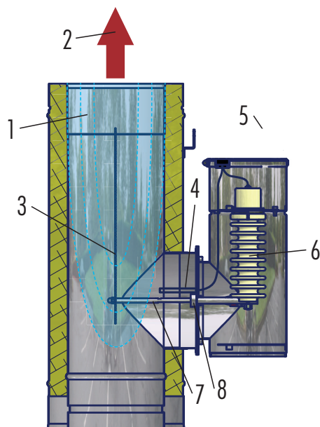
Abb. 10: Baugruppenübersicht Abscheidereinsatz (eingebaut in T-Stück DW)
