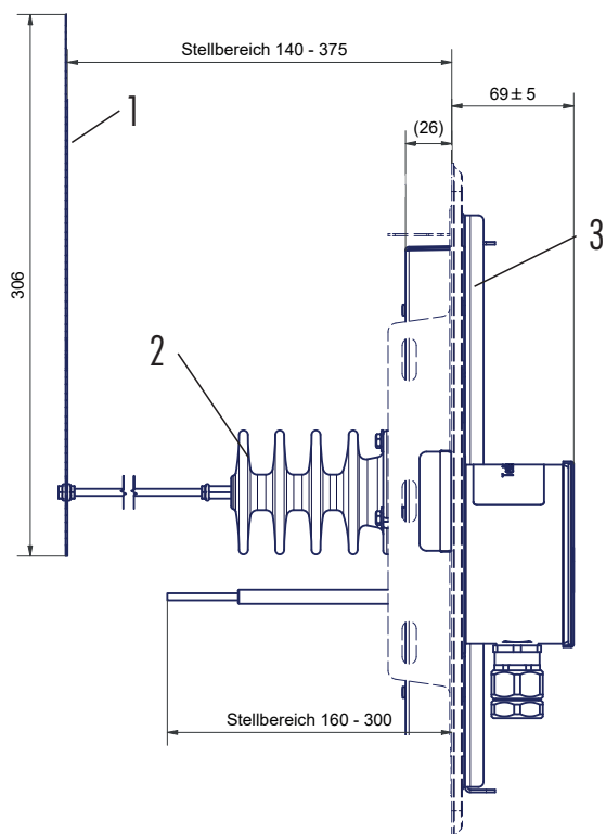
Abb. 22: Maße Zumikron® Ceramic mit Verschlussriegel 200x300, Elektrode (1), Keramikisolator (2), Putztüre (3)
