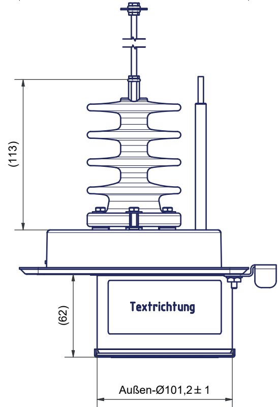
Abb. 7: Maße Ansicht 3 Partikelabscheider Zumikron® Ceramic mit Verschlussriegel 140x200 (Draufsicht)
