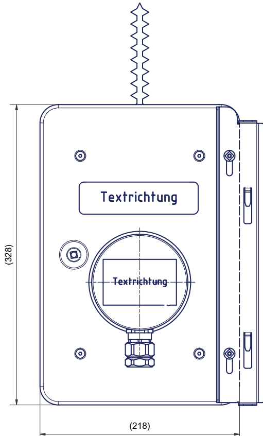
Abb. 9: Maße Ansicht 1 Partikelabscheider Zumikron® Ceramic mit Verschlussriegel 200x300 (Frontalansicht)
