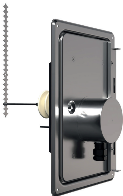
Abb. 20: Abscheidereinheit mit Putztür in Reinigungsverschluss- Rahmen montiert
