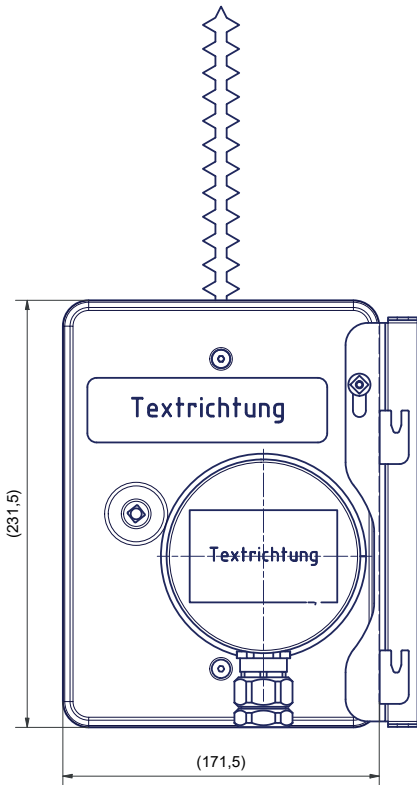
Abb. 5: Maße Ansicht 1 Partikelabscheider Zumikron® Ceramic mit Verschlussriegel 140x200 (Frontalansicht)
