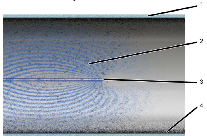
Abb. 17: Funktion Elektrostatische Partikelabscheidung
