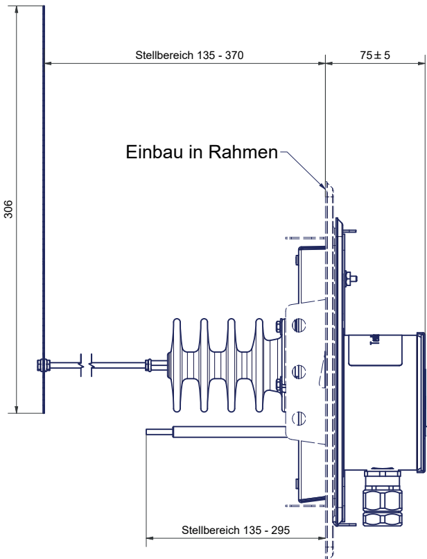
Abb. 6: Maße Ansicht 2 Partikelabscheider Zumikron® Ceramic mit Verschlussriegel 140x200 (Seitenansicht)
