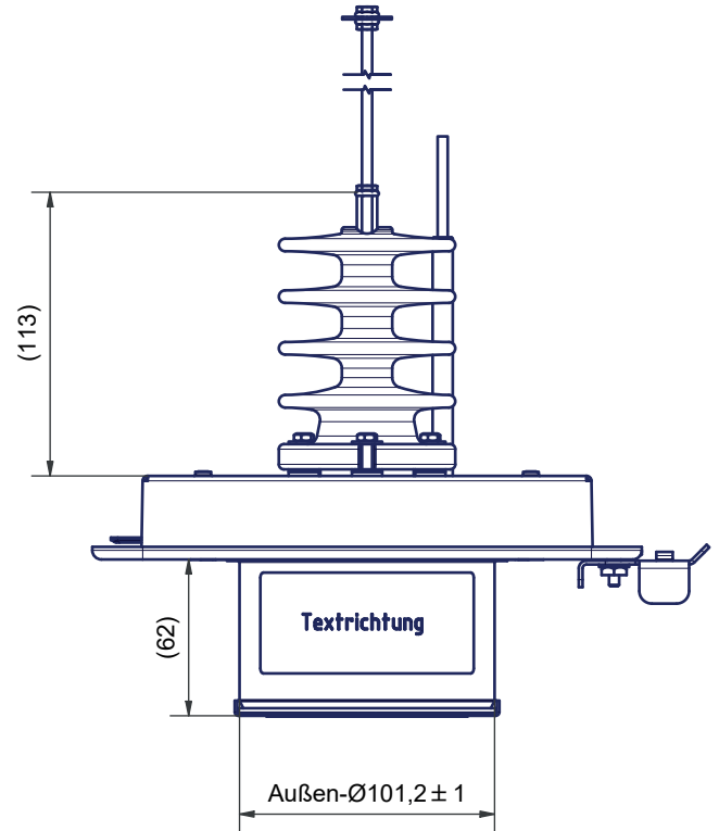
Abb. 11: Maße Ansicht 3 Partikelabscheider Zumikron® Ceramic mit Verschlussriegel 200x300 (Draufsicht)
