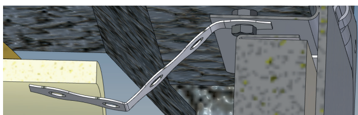
Abb. 23: Einbaubeispiel bei kurzem Türrahmen
