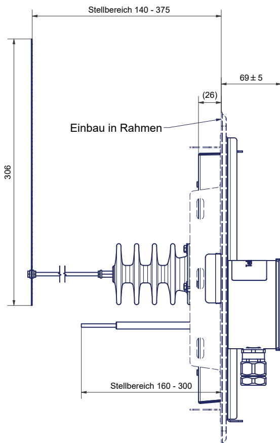
Abb. 10: Maße Ansicht 2 Partikelabscheider Zumikron® Ceramic mit Verschlussriegel 200x300 (Seitenansicht)
