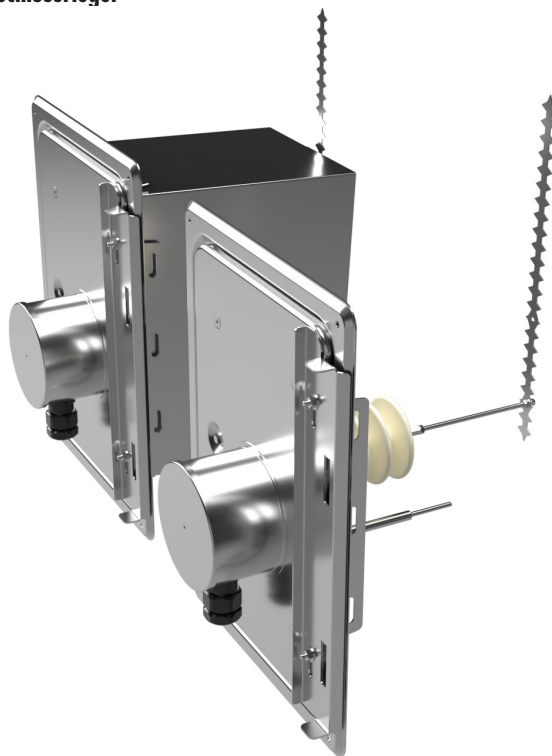
Abb. 18: Abscheidereinsatz in Putztürrahmen montiert (rechts) Abscheidereinsatz in Putztürrahmen mit verlängertem Schacht (links)
