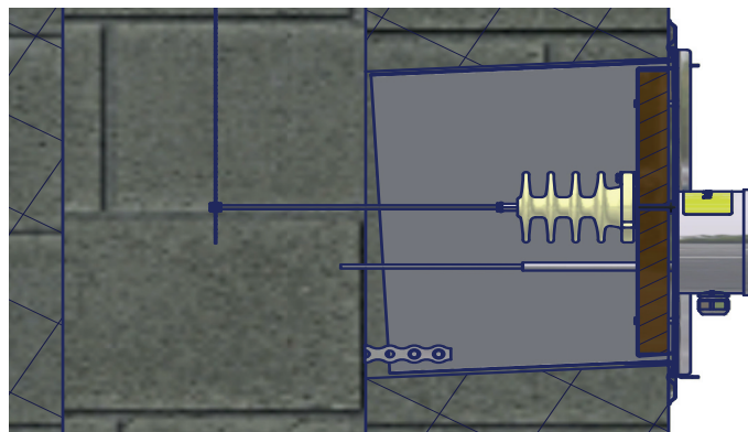
Abb. 24: Einbaubeispiel bei verlängerter Putztüre
