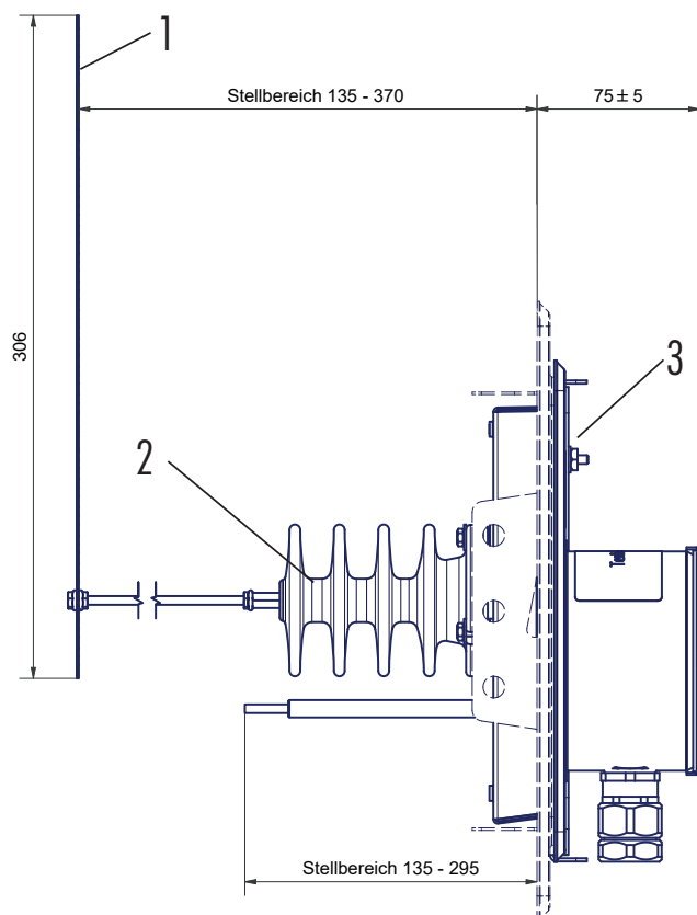
Abb. 21: Maße Zumikron® Ceramic mit Verschlussriegel 140x200, Elektrode (1), Keramikisolator (2), Putztüre (3)
