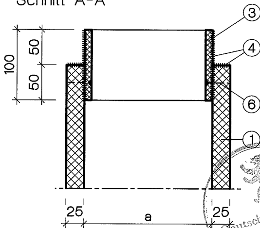
Schnitt A-A
