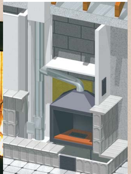
Beispielanwendung für einen offenen Kamin
