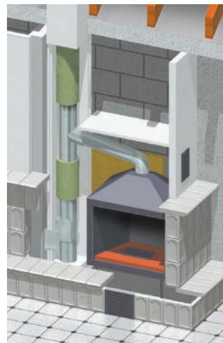
Beispielanwendung für einen offenen Kamin
